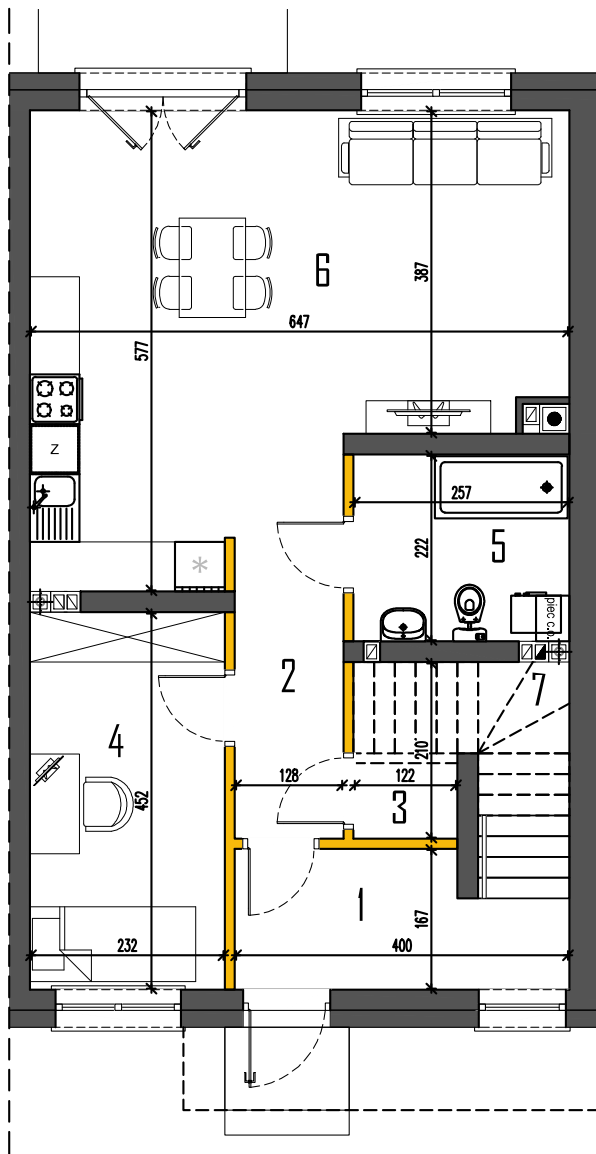
RZUT PARTERU
