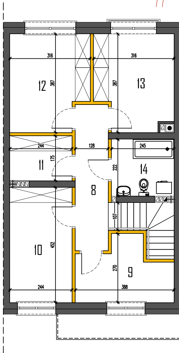
RZUT PIĘTRA
